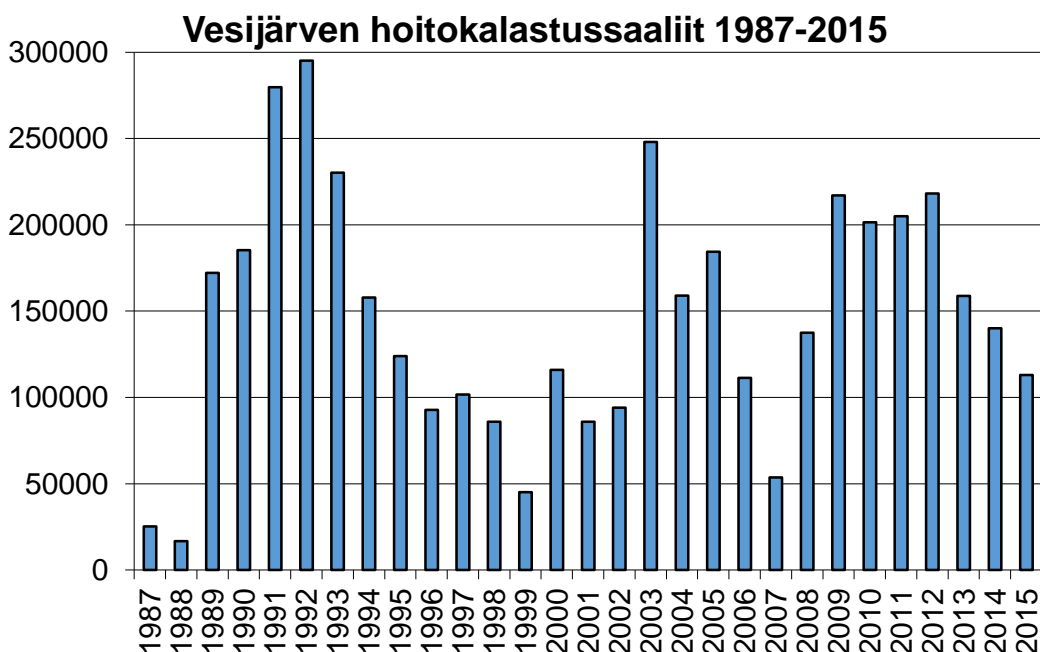
Kuva 1. Vesijärven hoitokalastussaaliit 1987-2015
